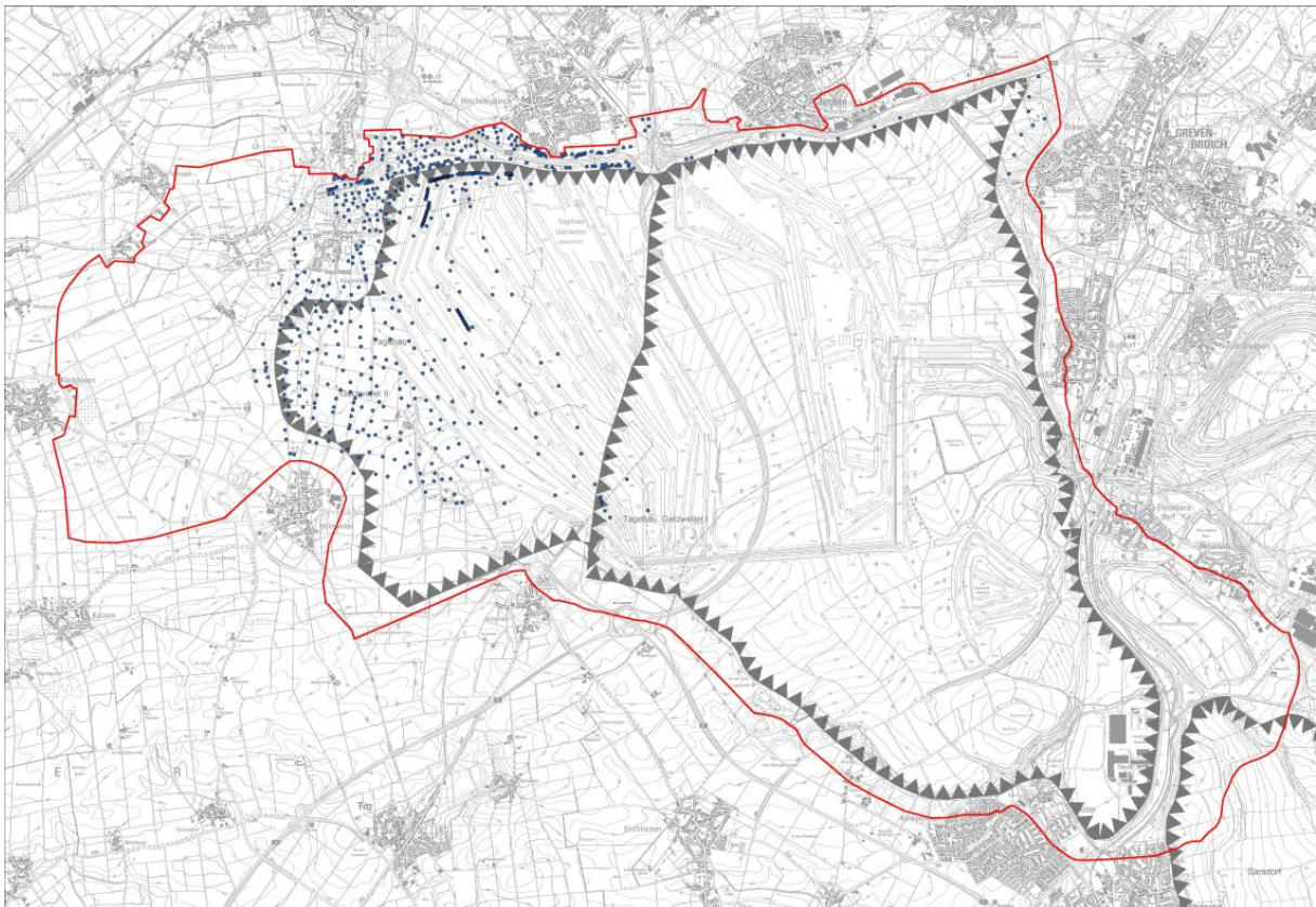
Abbildung 5: Aktueller Grundwasserentnahmebereich sowie Lage der aktiven Brunnen. (UP/UVP-Angaben 2025).
