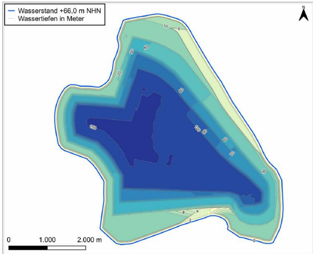
Abbildung 9: Geometrie inkl. Wassertiefen des Tagebausees Garzweiler II bei Erreichen des Zielwasserspiegels i. H. v. +66 m NHN (BTU Cottbus-Senftenberg, RWTH Aachen, IWB Dr. Uhlmann & IfB Potsdam-Sacrow 2025). (Quelle: UP/UVp RWE Power AG, 2025).
